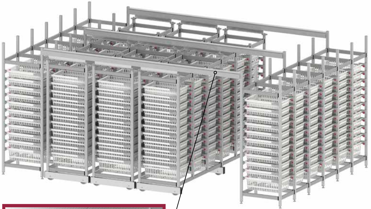
Esempio di scaffalatura compattabile tipo "UUU"
